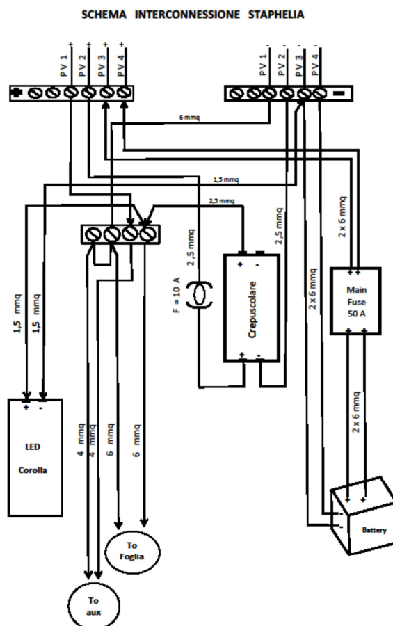
Figura 21: Schema alimentazione
