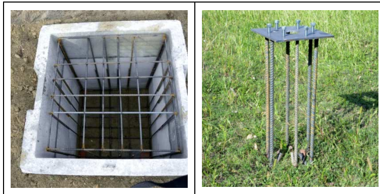
Figura 18: il plinto
